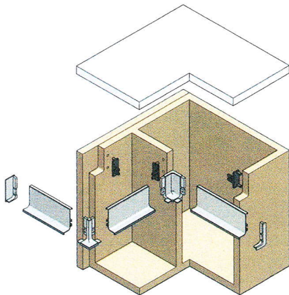
horizontálny dvierkový "J" profil
