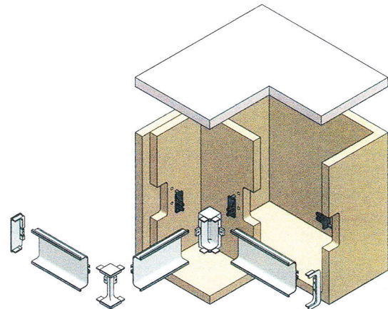
horizontálny zásuvkový "C" profil
